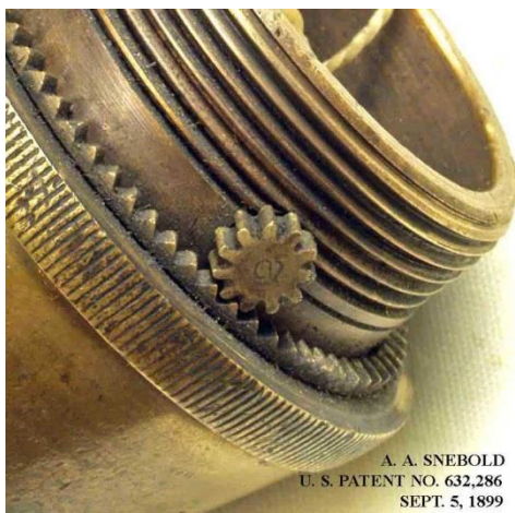
A. A. SNEBOLD U. S. PATENT NO. 632,286 SEPT. 5, 1899
